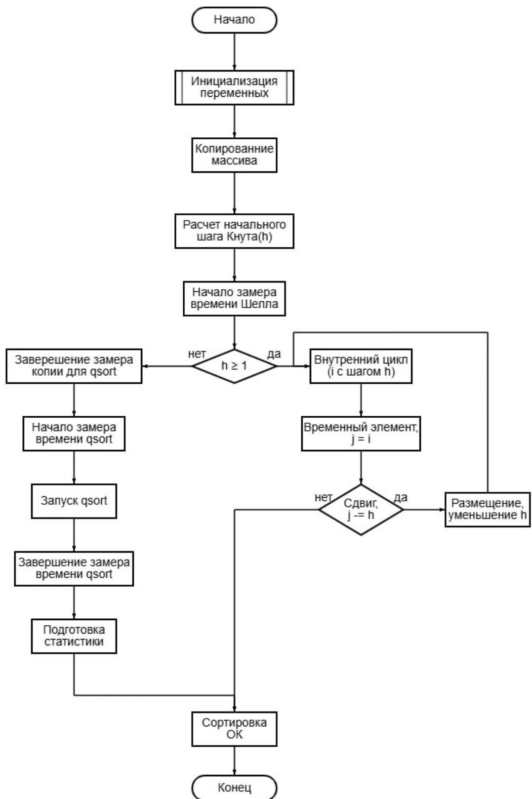
Рисунок 2 - Блок-схема алгоритма сортировки
