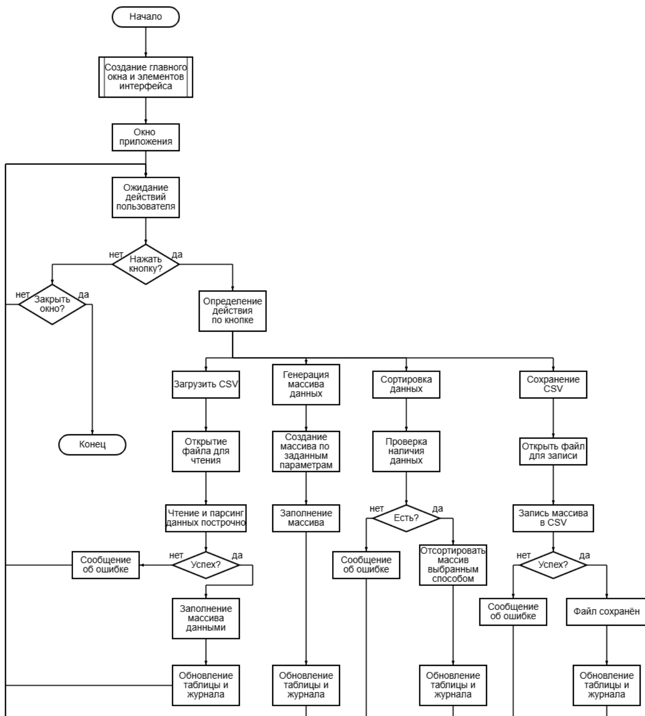
Рисунок 1 - Блок-схема программы
